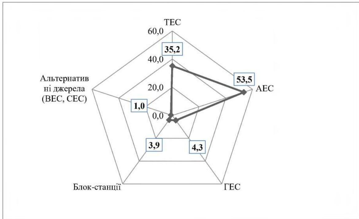
Рис. 3.12. Структура виробництва електроенергії по ОЕС України в середньому упродовж 2015–2018 рр., %
